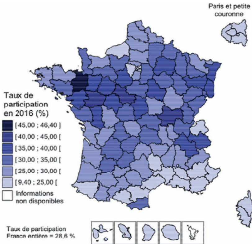
FIGURE 5. Variation du taux de participation de la population selon les départements (période 14 avril 2015 – 31 décembre 2016). Données : Santé Publique France, février 2017 (traitement INCa, mai 2017).
